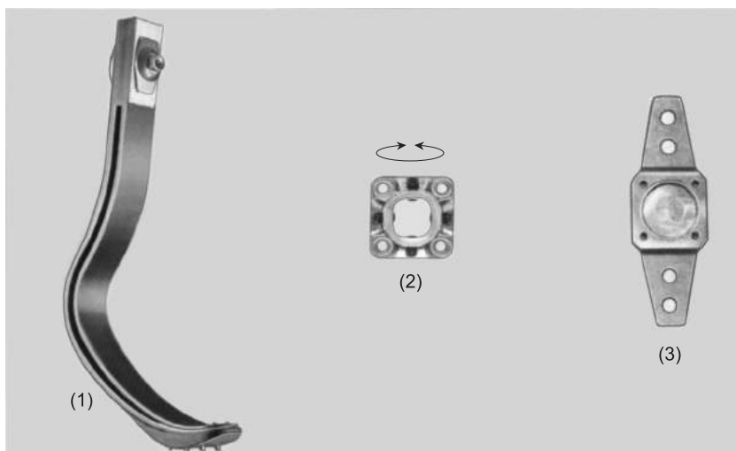
Рис. 6. Стопа ОТТО-ВОСК C-Sprint (1) с адаптером (2) и юстировочным элементом (3)
