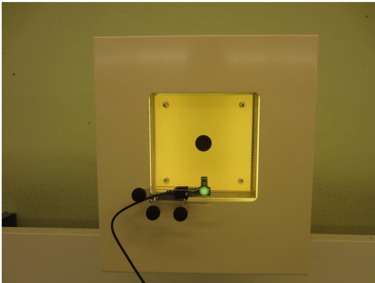
Пример универсального ИК-блока, установленного на мишени Meyton, который питается от USB.
